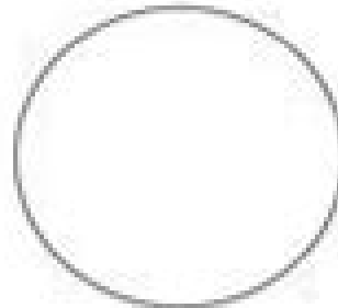
Venus
