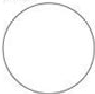
Earth
