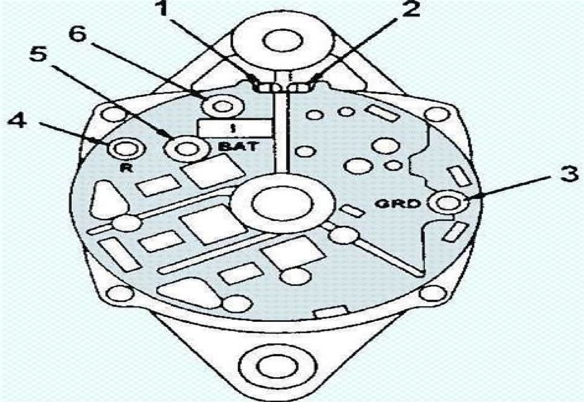
Трехфазный генератор Delco-Remy: 1, 6 - контрольная лампа; 2 - вывод для измерения напряжения; 3 - вывод на массу; 4 - индикатор; 5 - вывод на аккумулятор
