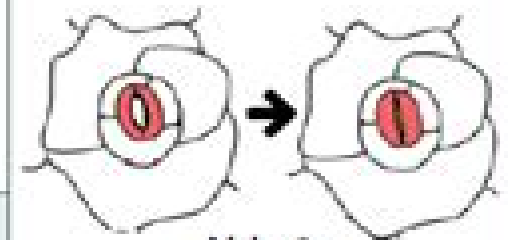
Abb. 2: Spaltöffnungen
