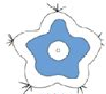
Abb. 3: Wasserspeicherung
