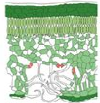
Abb. 1: verdickte Blätter
