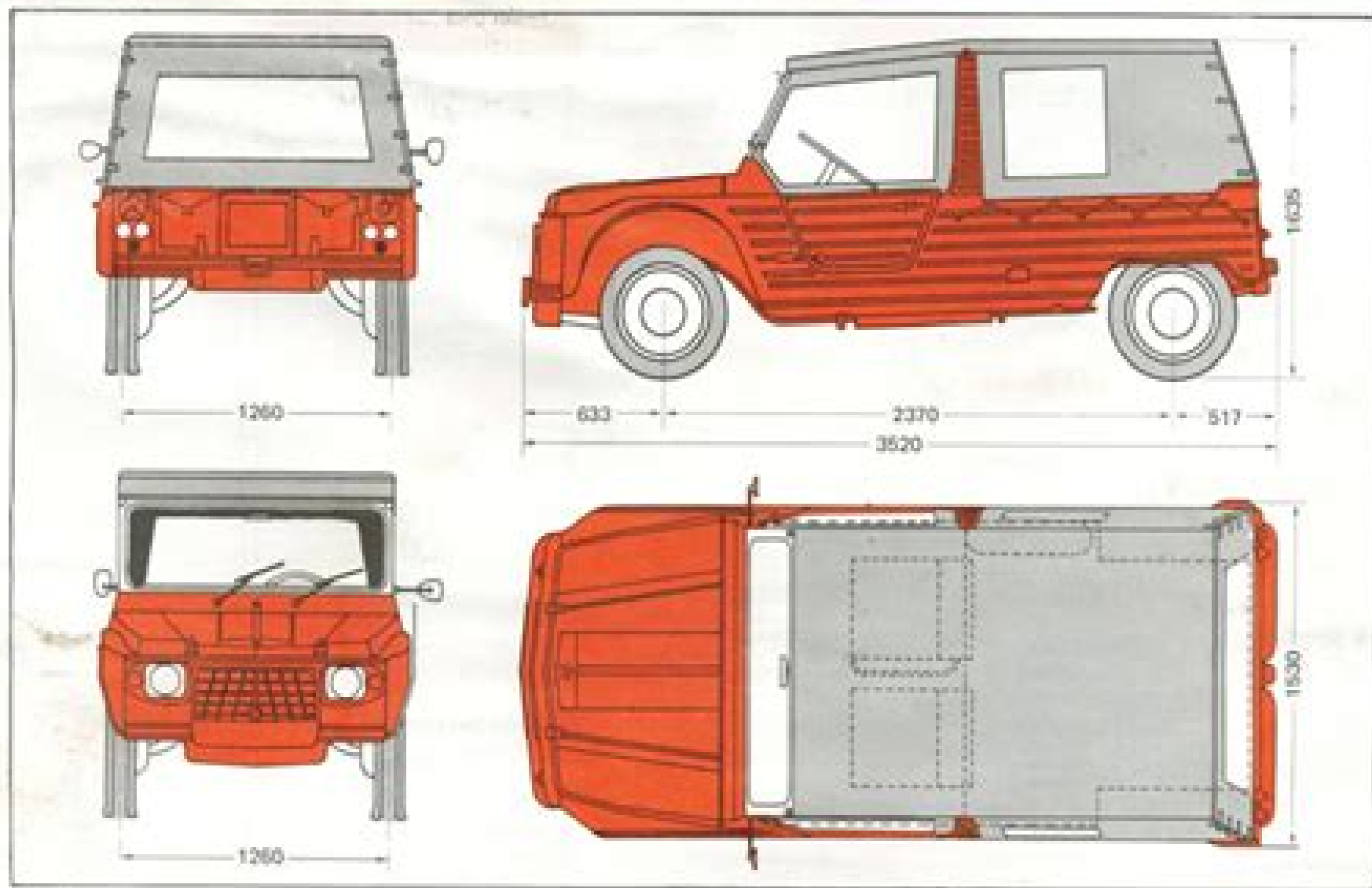
Fig. 57 - Cotas de las dimensiones
