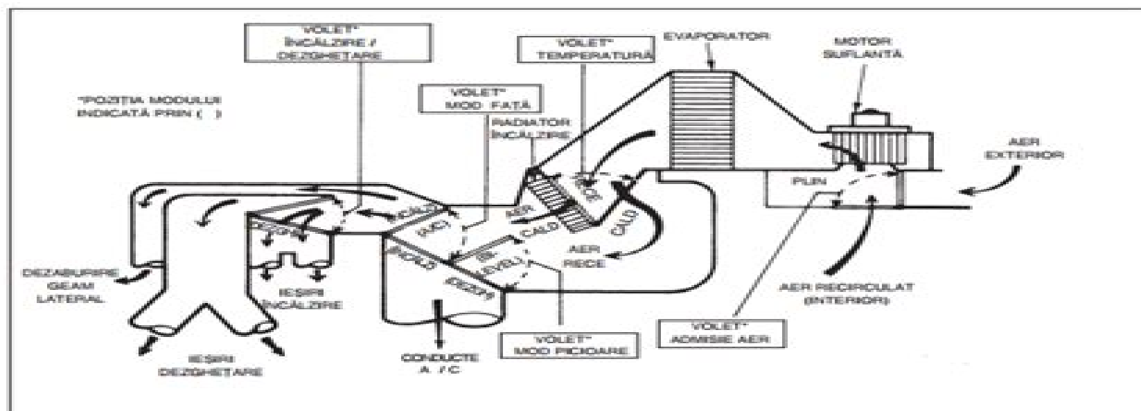
Fig. 3 Schemă curgere aer
