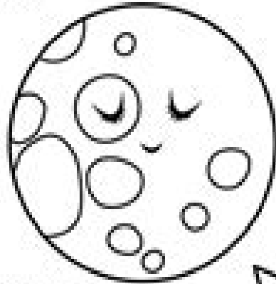
MOON
