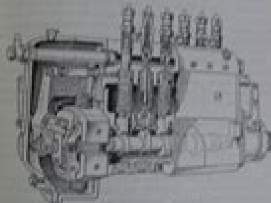
Fig. 102. Het mechanisme van de continuïteit regulator, dat in zijn werking het werk van de regulator, het mechanisme R.
