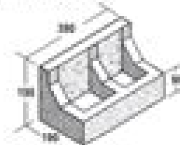
20.45 Header
