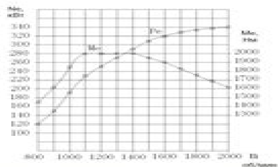
Рис. 2. Внешняя скоростная характеристика дизельного двигателя D12.46-30
