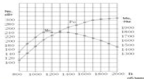
Рис. 3. Внешняя скоростная характеристика дизельного двигателя D12.42-30
