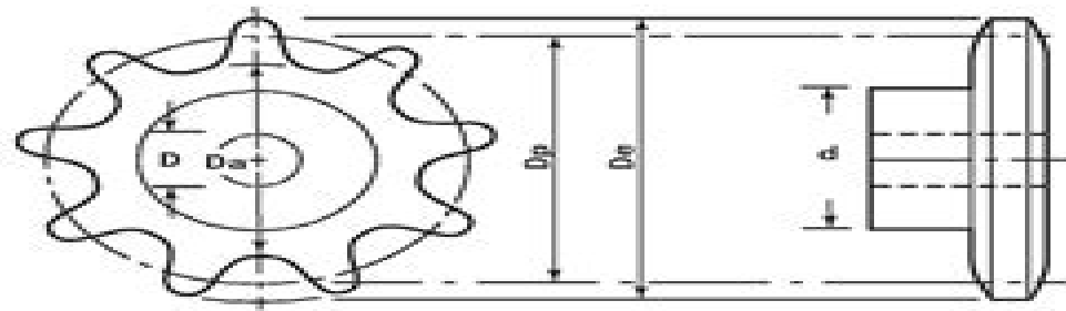
Sprocket Diameters
