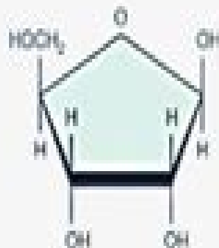
RIBOSE
