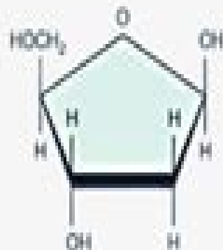
DEOXYRIBOSE
