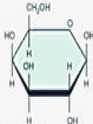
GALACTOSE
