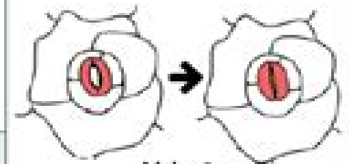
Abb. 2: Spaltöffnungen
